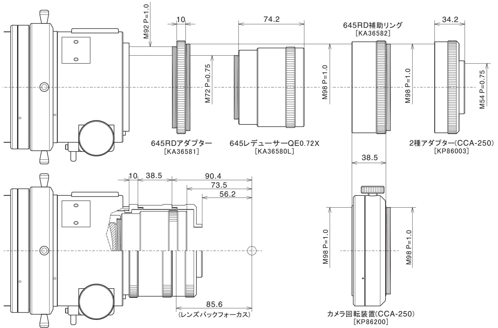
645レデューサーQE0.72X寸法図面 2011/09/08 (株)高橋製作所
